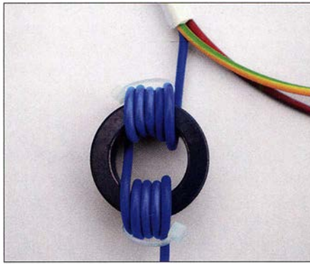
Bild 4: Für die Ringkerndrosseln auf der Primärseite empfiehlt sich das gleiche Wickelschema wie auf der Sekundärseite.
