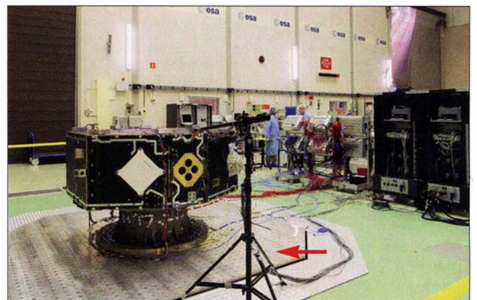
Bild 7: Das STM (engl. structural thermal model ) des LISA Pathfinder ist hier für einen Vibrations-test auf dem Quad Multishaker montiert.
