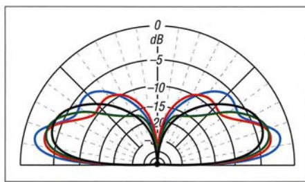
Bild 4: Simulierte Strahlungsdiagramme des Vertikaldipols mit 2 x 7 m über realem Grund ( \epsilon_r = 13, \sigma = 5 \text{ mS/m} ) bei 18,1 MHz (blau), 14,5 MHz (rot), 10,1 MHz (grün) und 7,1 MHz (schwarz); äußerer Ring 0 dB \hat{=} 1,45 \text{ dBd}
