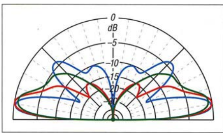
Bild 3: Simulierte Strahlungsdiagramme des Vertikaldipols mit 2 x 7 m über realem Grund ( \epsilon_r = 13, \sigma = 5 \text{ mS/m} ) bei 28,5 MHz (blau), 24,9 MHz (rot) und 21,2 MHz (grün); äußerer Ring 0 dB \hat{=} 1,45 \text{ dBd}
