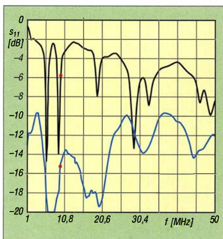
Bild 7: Gemessene Reflexionsdämpfung der AS2599 (schwarz) im Vergleich zum bedämpften Breitbanddipol (blau); die Marker zeigen bei 9,96 MHz die Werte S_{11} = -5,5 \text{ dB} ( s = 3,3 ) bzw. S_{11} = -14,9 \text{ dB} ( s = 1,4 ).
