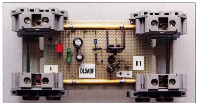
Bild 6: Aufbau der Überspannungssicherung auf einer Lochrasterplatine
