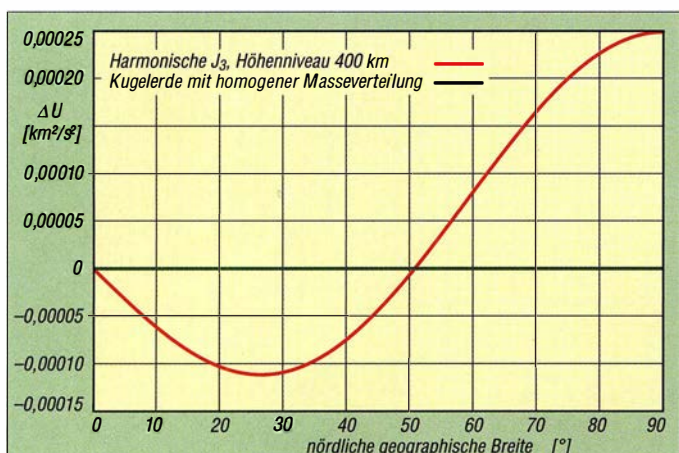
Bild 8: Die „Birnenform“ der Erde: Differenz im Gravitationspotenzial \Delta U zwischen Nord- und Südhalbkugel im Höhengiveau der ISS, in Bild 6 noch nicht erkennbar
