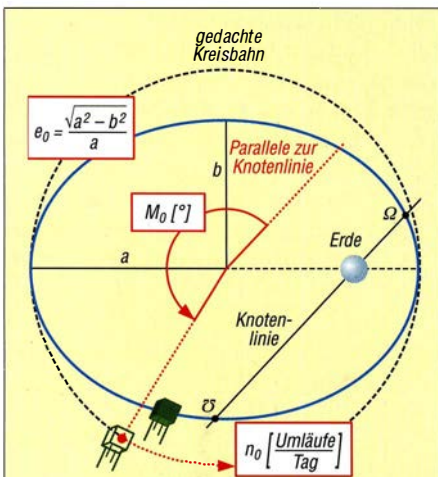
Bild 3: Blick senkrecht auf die Bahnebene; der Satellit umrundet die Erde auf einer Kreisbahn mit konstanter Winkelgeschwindigkeit. Dann beschreiben die Bahnelemente mittlere Anomalie M_0 dessen Ort, mittlere Bewegung n_0 dessen Geschwindigkeit. Exzentrizität e_0 definiert die Form der Bahnellipse, alles zur Epochezeit.
