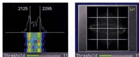
Bilder 12 und 13: Die beiden Abstimmhilfen für RTTY-Betrieb (FSK)
