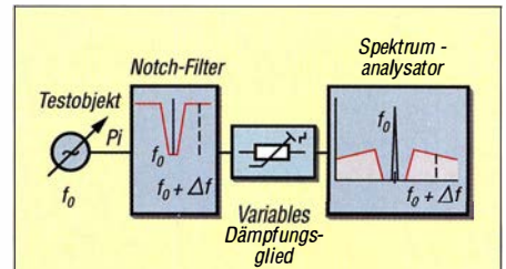
Bild 22: SBN-Messung eines Oszillators mithilfe eines Notch-Filters
