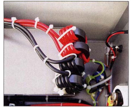
Bild 5: Die parallelgeschalteten Kabel auf der Sekundärseite des Schaltnetzteils erhöhen den wirksamen Leiterquerschnitt.
