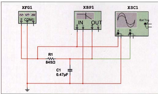
Bild 9: RC-Tiefpassfilter mit Funktionsgenerator (links), Bode-Plotter (Mitte) und Oszilloskop (rechts)
