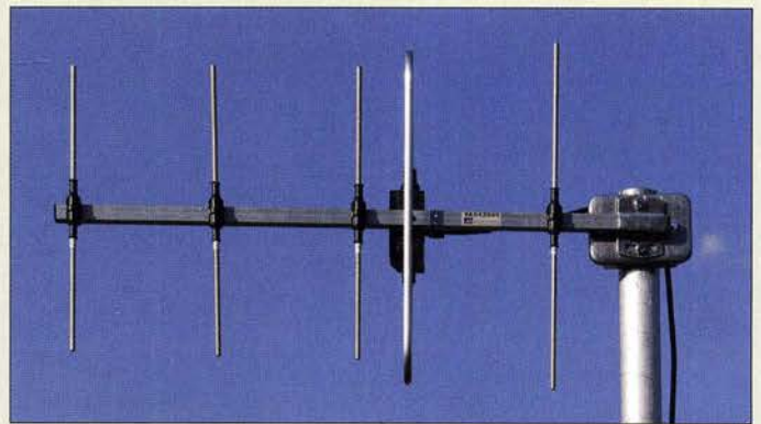
Yagi-Antenne YA043505E in Vormastmontage
