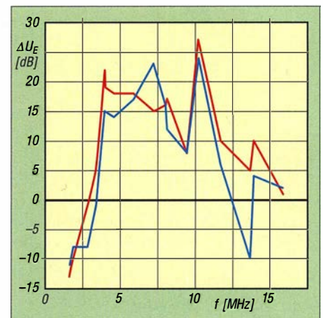
Bild 8: Pegeldifferenzen im Empfangsvergleich zwischen AS2599 (blau) bzw. Breitbanddipol (rot) und Aktivantenne (Referenz)
