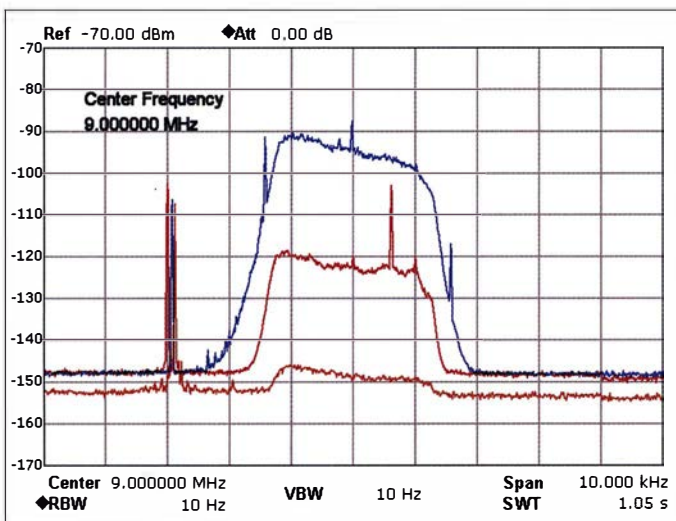
Bild 21: Seitenbandrauschen des Signalgenerators Marconi 2019, gemessen mithilfe eines Notch-Filters; Noise-Marker 1 liefert -129,8 dBm/Hz Foto und Screenshots: DC4KU
