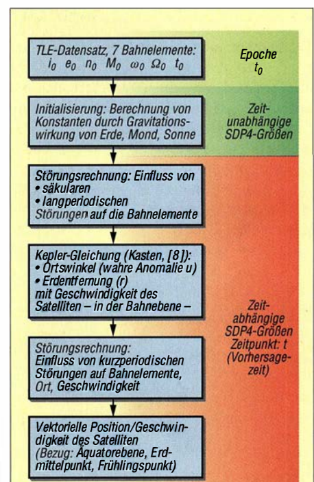
Bild 5: Vereinfachtes Rechenschema des SDP4-Modells; alle Störeinflüsse durch Erde, Sonne und Mond sind im Modell rein gravitativer Natur.
