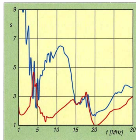
Bild 4: Stehwellenverhältnisse an der 5,5 m langen Antenne bei Verwendung eines 1:16-Unun ohne (blau) und mit 820-Ω-Widerstand (rot)
